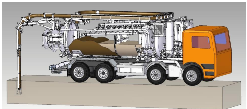
Flockungsprozess: Separierung des festen und flüssigen Saugguts
