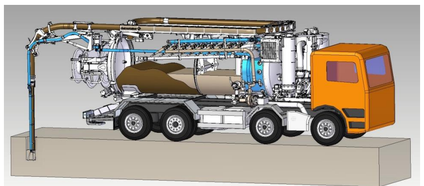
Rückführung des aufbereiteten Schachtwassers in den Strassenschacht, über einen separaten Rückgabeschlauch
