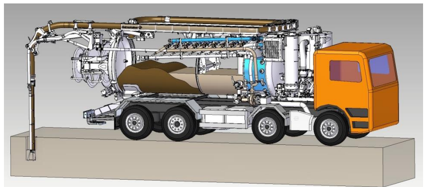
Feinfiltration und Weiterleitung des flüssigen Saugguts zum Wassertank
