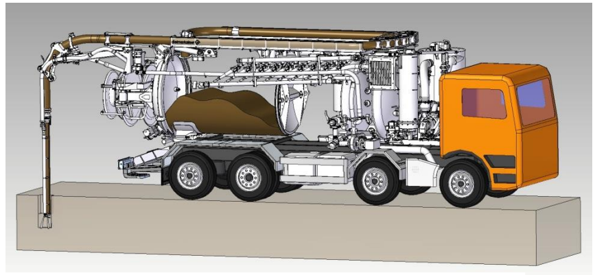
Aufnahme des Schachtmaterials in den Schlammtank
